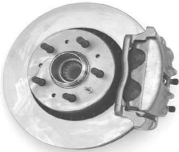
Girling 2-Kolben Bremssattel ohne ABS -1991 mit ABS -1990
